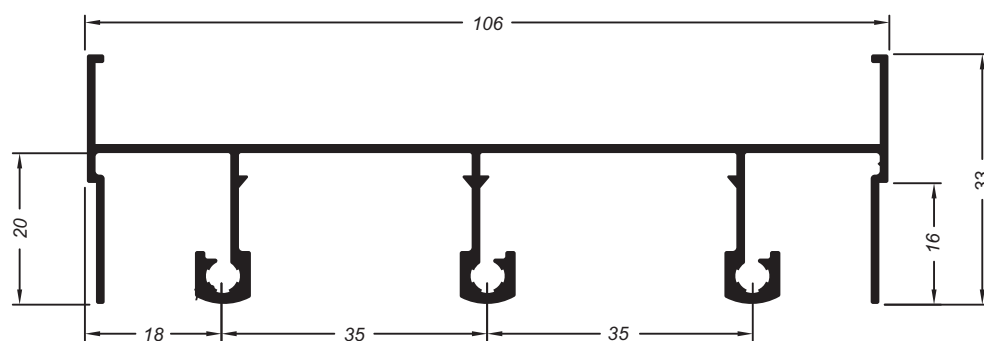
Trilho superior triplo
