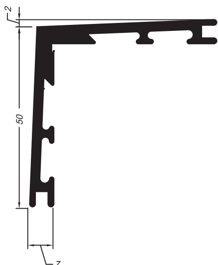
Cantoneira cunha (conexão)
