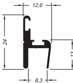
Cadeirinha 8mm
