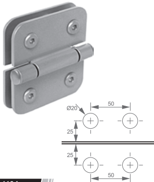
1134 /// Dobradiça MAXIM-AR V/V 50mm entre furos
