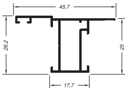
Montante travessa 45 graus
