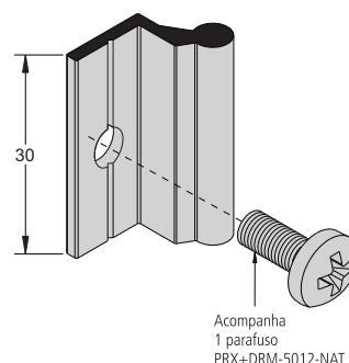
Presilha de fixação dos quadros
