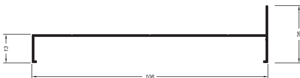
Trilho superior triplo
