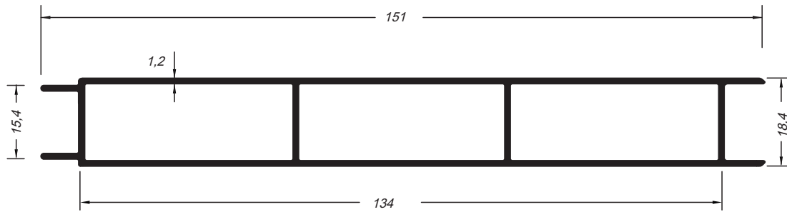
Lambril da porta
