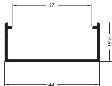
MK-79 Corrimão encaixe inferior 0,311 Kg/m
