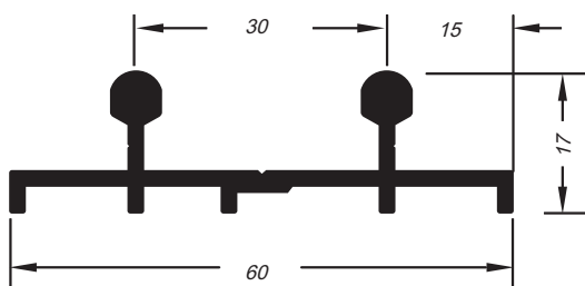
Trilho superior guia deslizante
