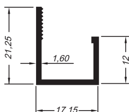
Capa sacada inferior
