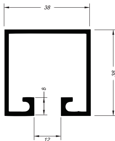
Trilho Sanley 38 e 38mm MK-37 0,717 Kg/m
