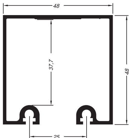
Trilho Sanley 48 e 48mm
