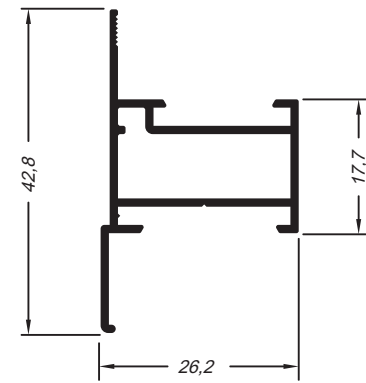
Montante da folha
