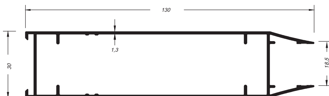
Montante porta 130 mm PT-303 1,299 Kg/m
