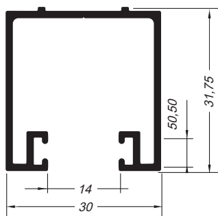
Trilho superior guia deslizante
