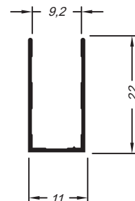
Baguete (cavalinho) U perfil fixo 8mm
