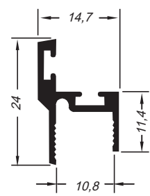
Cadeirinha 10mm leve
