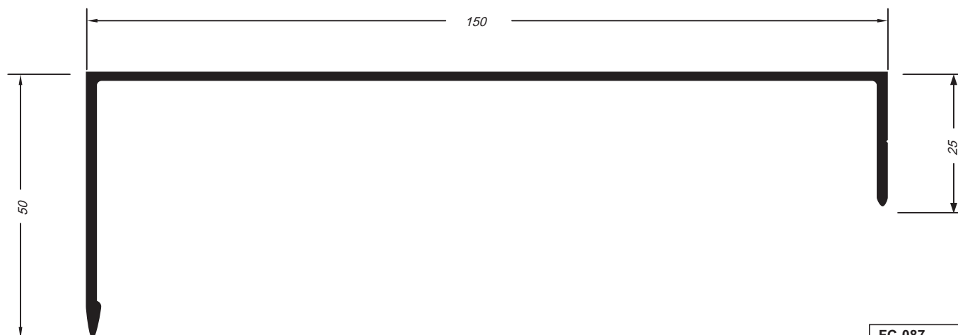
Acabamento lateral
