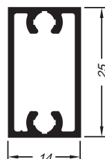
Tubo pontaleta sacada
