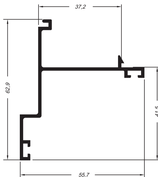
Travessa fixa
