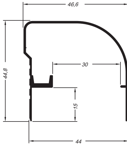
Trilho superior redondo MK-86 0,440 Kg/m
