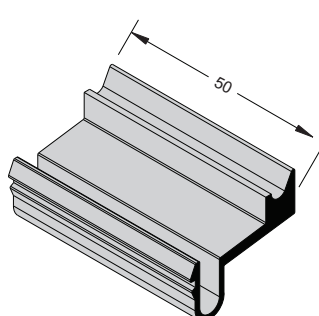
Presilha de apoio dos quadros
