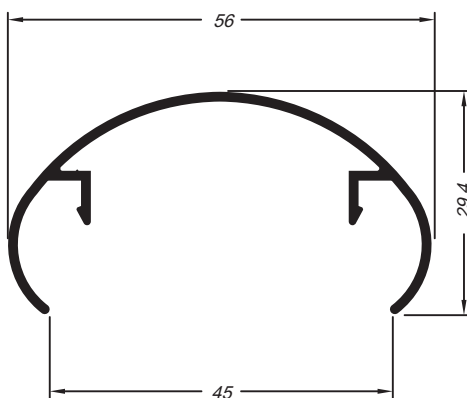
MK-78 Corimão encaixe superior 0,409 Kg/m
