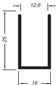
Baguete (cavalião) U 10mm
