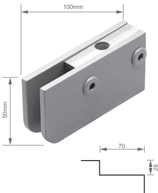
1101M /// Dobradiça superior mini
