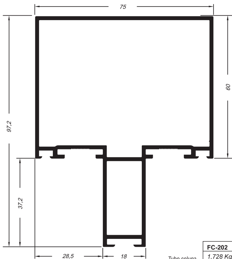
Tubo coluna
