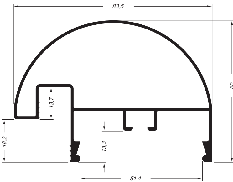
MK-84 Corrimão sacada redondo 1,077 Kg/m
