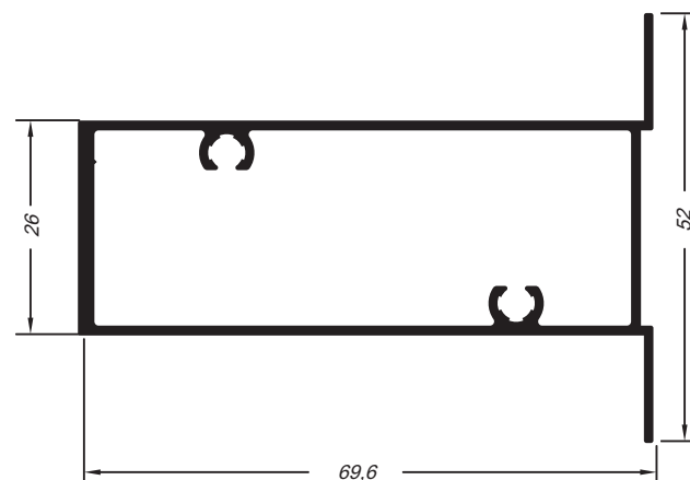
Marco da bandeira
