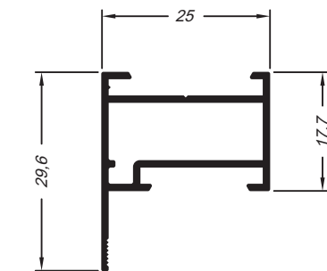
Travessa superior da folha
