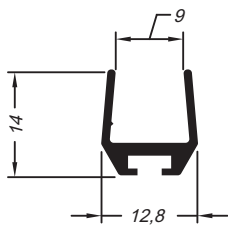
Transpasse vedação 8 e 10mm
