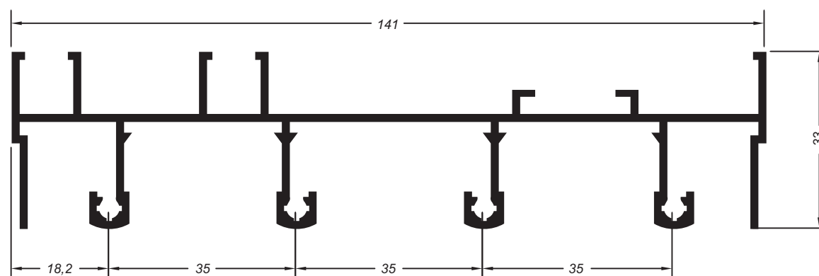
Marco lateral 4 folha
