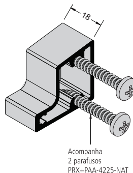
Fixador de travessa para FA-211/FA-233
