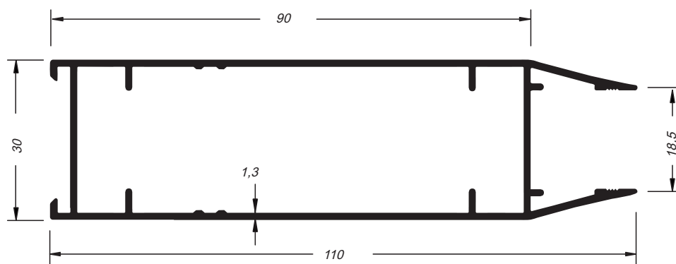
Montante porta 110 mm PT-304 1,152 Kg/m
