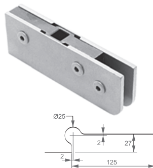
1103 /// Dobradiça interior c/ encaixe p/ mola
