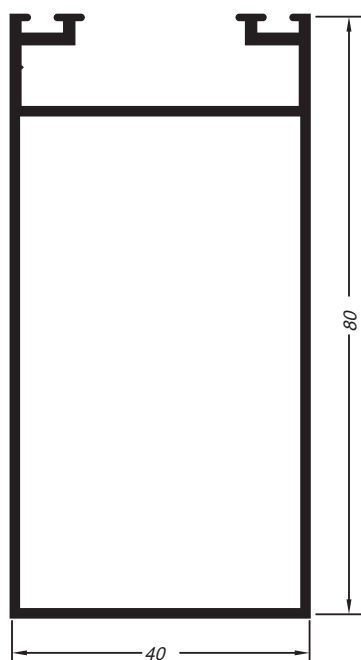
Tubo coluna
