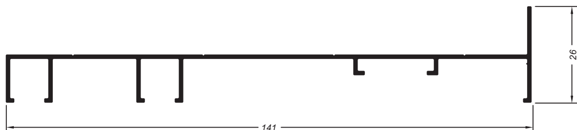
Marco lateral para 3 folha
