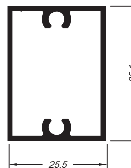
Perfil J para vidro fixo sacada
