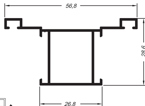
Coluna travessa
