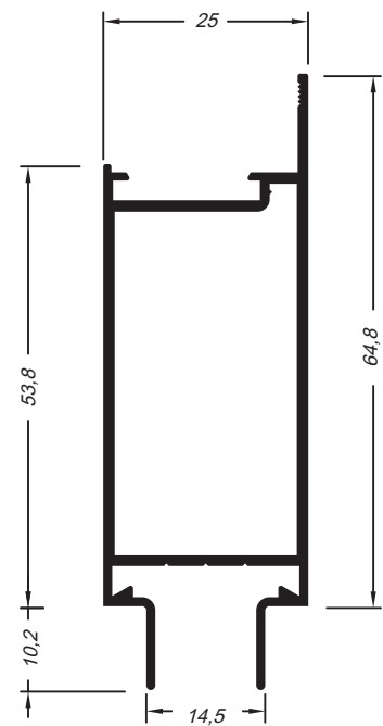
Montante mão amiga porta
