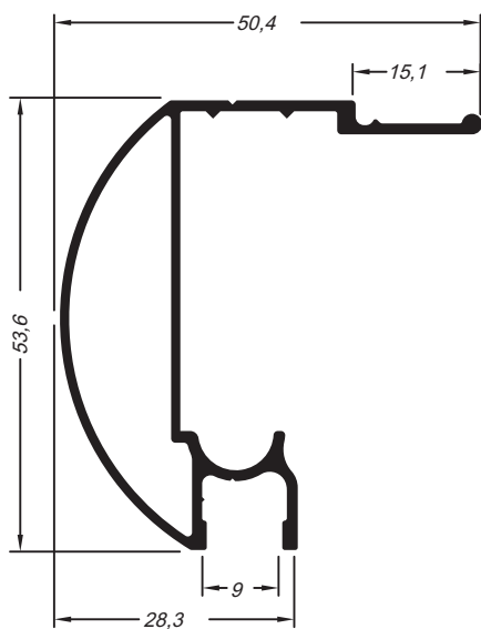
Trilho superior box 8mm temp. MK-60 0,612 Kg/m
