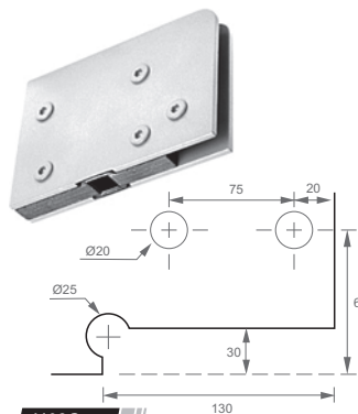
1103G /// Dobradiça interior grande c/ encaixe p/ mola
