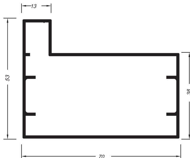
Tubo vista lateral
