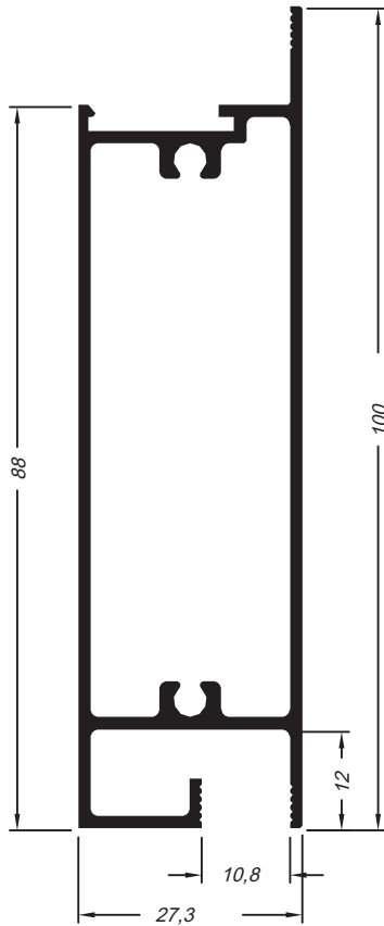
Travessa montante da folha
