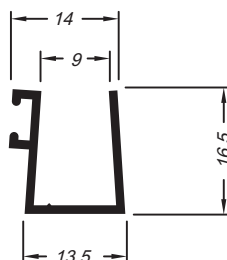
Transpasse 8 e 10mm
