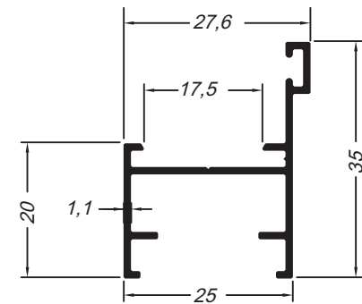
Travessa superior da folha
