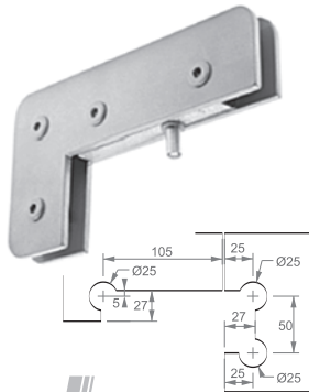
1209 /// Facão simples p/ lateral e bandeira
