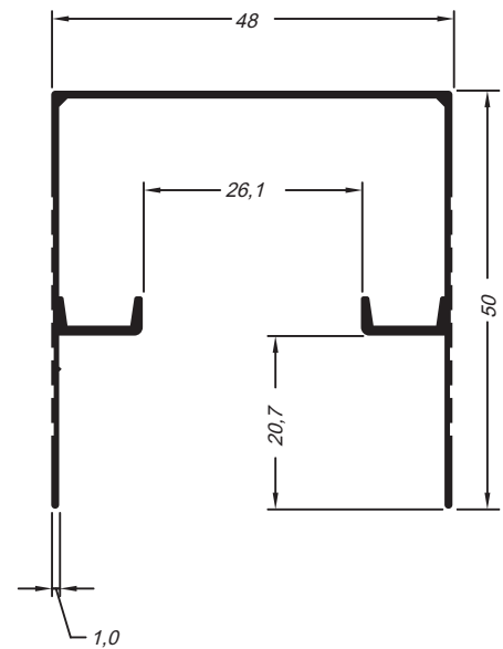
Trilho superior quadrado duplo MK-157 0,466 Kg/m
