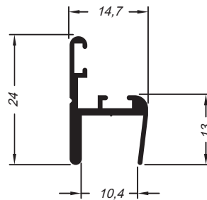
Cadeirinha 10mm leve
