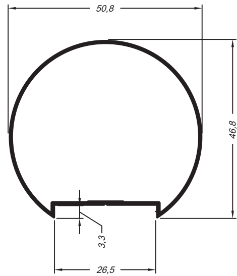
MK-71 Corrimão redondo 0,493 Kg/m
