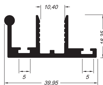
Mão amiga deslizante
