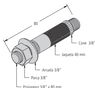
Chumbador expansivo sem prolongador 3/8" x 80mm
