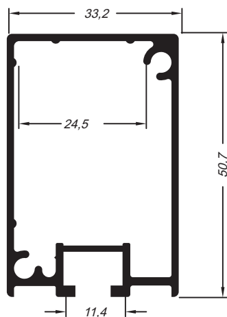
Tubo pontaleta sacada
