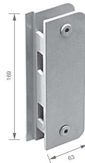
1504TAF /// Contra fechadura V/V s/ furo p/ 1520TA
