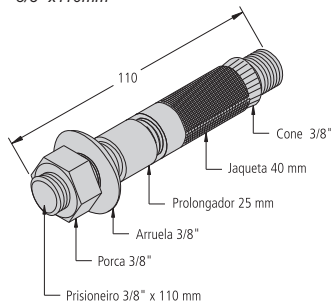
Chumbador expansivo com prolongador 3/8" x 110mm
