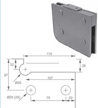
1101G /// Dobradiça superior grande
