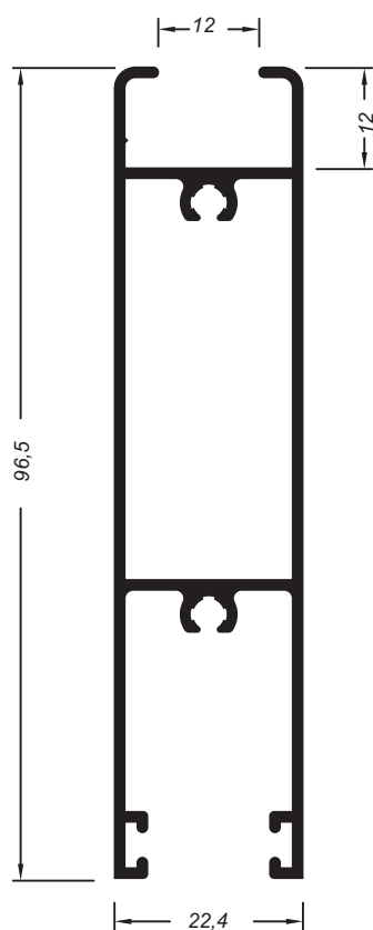
Montante mão amigo puxador tubular
